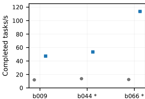
YOLOv7 / H8
