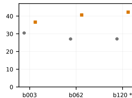
YOLO26m / H10
