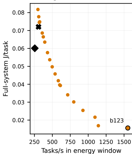
RegNetX-1.6GF / H10
