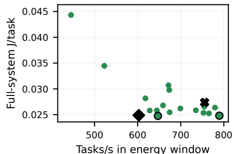
RegNetX-1.6GF / DeepX
