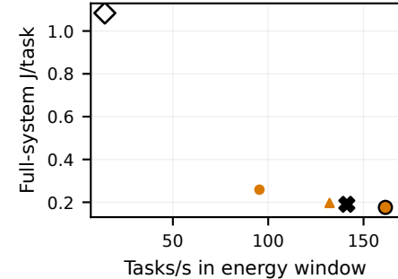
YOLOv7 / H10
