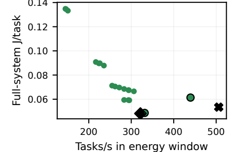
YOLO11l / DeepX
