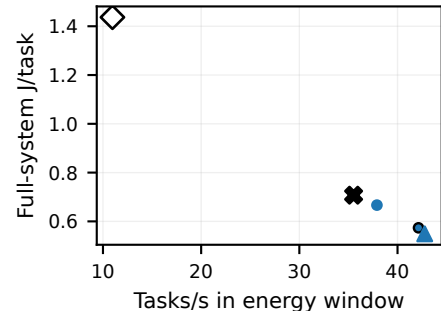
YOLO26m / H8
