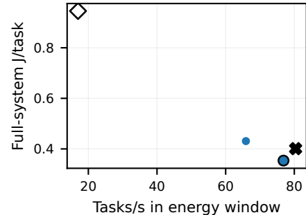
YOLO26s / H8
