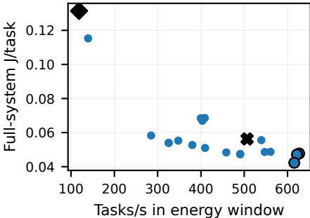
YOLO11l / H8
