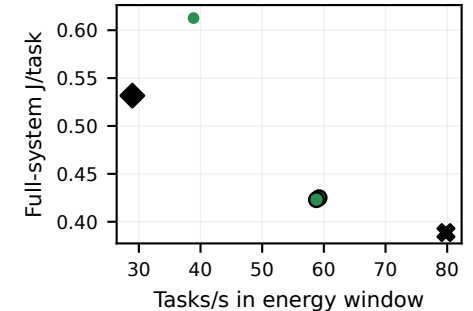
YOLO26s / DeepX
