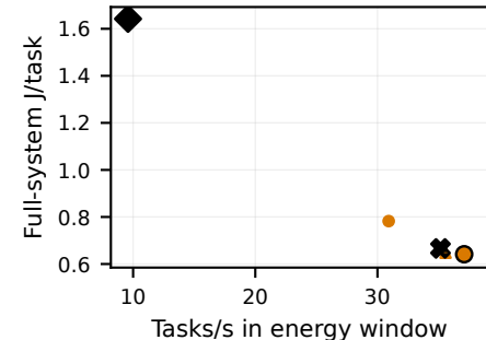
YOLO26m / H10
