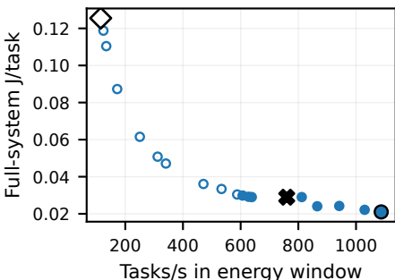
RegNetX-1.6GF / H8
