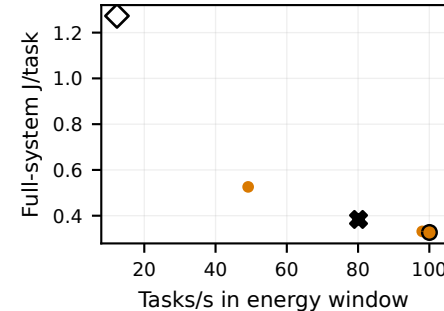
YOLO26s / H10
