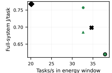
YOLO26m / DeepX
