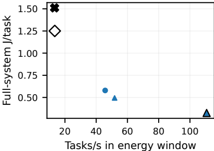
YOLOv7 / H8
