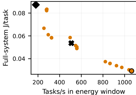
YOLO11l / H10
