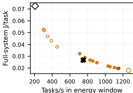
RegNetX-1.6GF / H10
