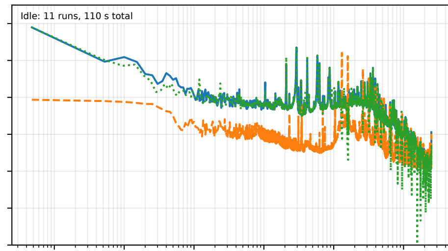
(d) YOLO-INT8
