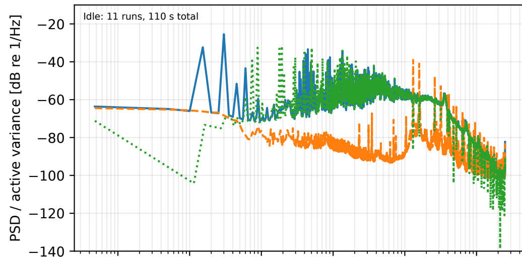
(e) Gemma3-4B
