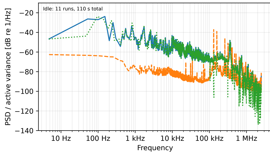
(e) Gemma3-4B
