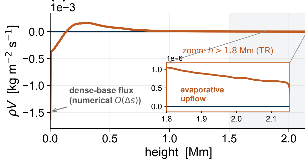
(d) Mass flow
