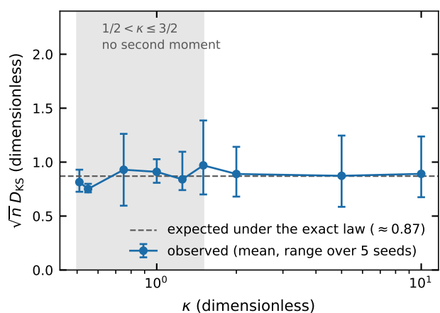
(d) radial KS statistic vs \kappa
