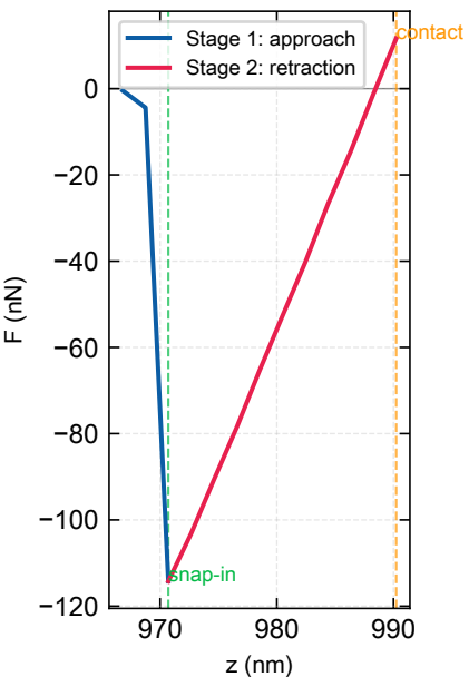
JJS-50nm-1500nm-10nN
