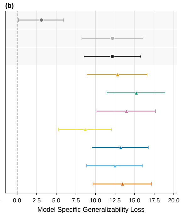
Evaluation: EUH
