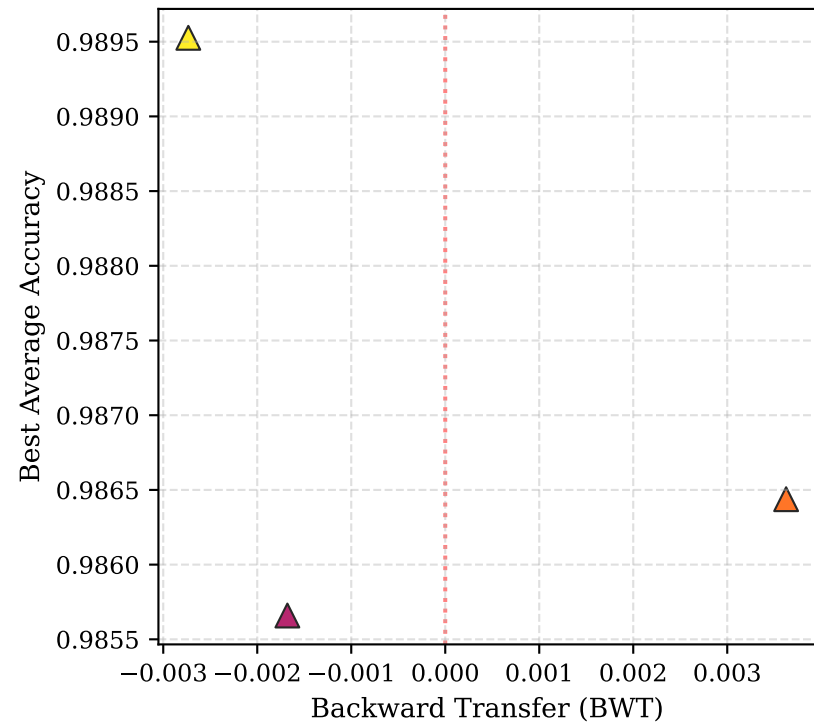
(a) Sweep A: split-MNIST
