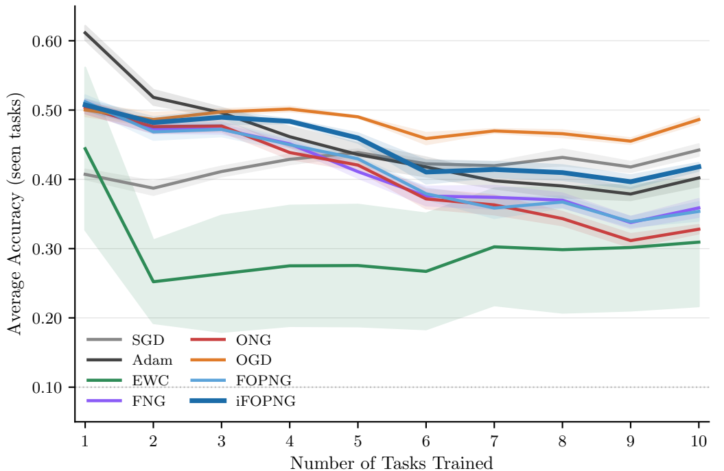
Split-CIFAR100
