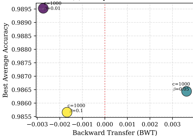
(a) Sweep A: MNIST SH
