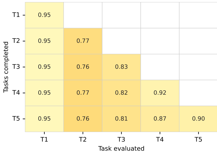
eFOPNG
