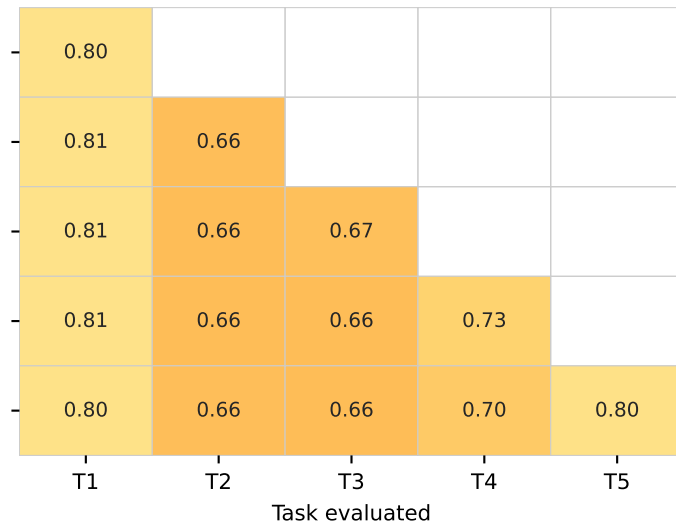
FOPNG
