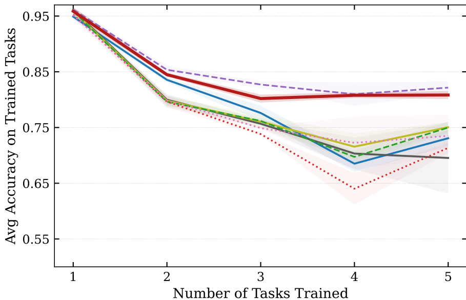
C4 · Split-CIFAR10 MH · Standalone
