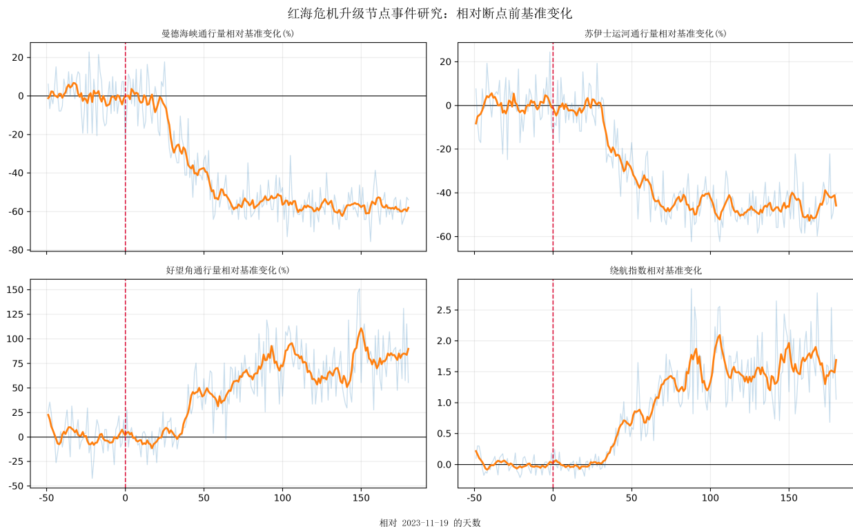
Figure 3: 2023-11-19 事件研究曲线
