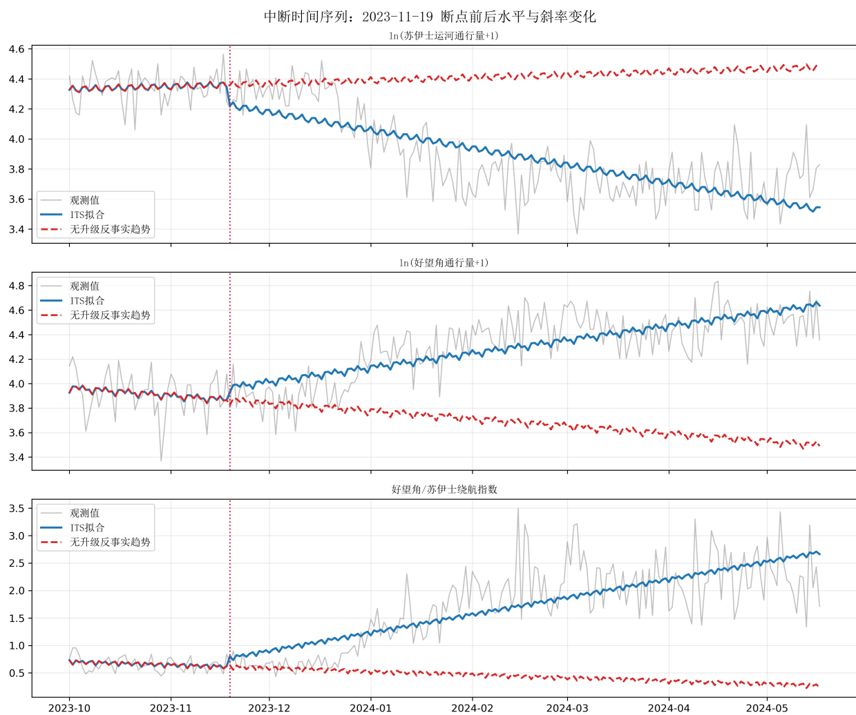
Figure 4: 中断时间序列拟合曲线
