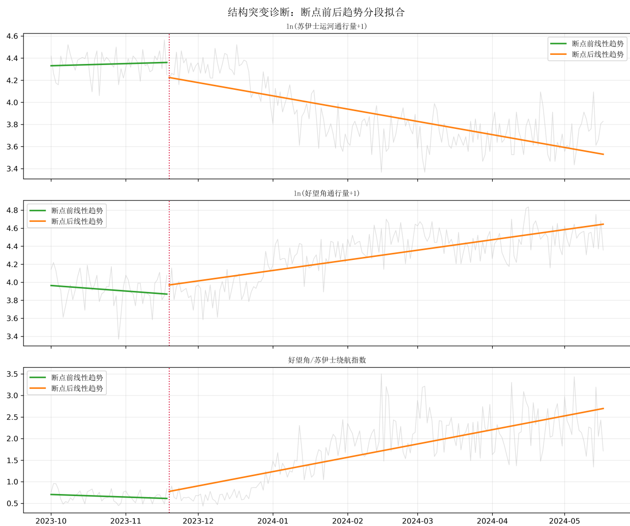
Figure 5: 结构突变诊断曲线
