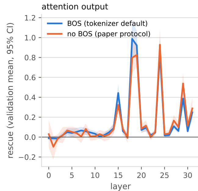
Mixtral-8x7B-v0.1: BOS vs no-BOS tokenisation
