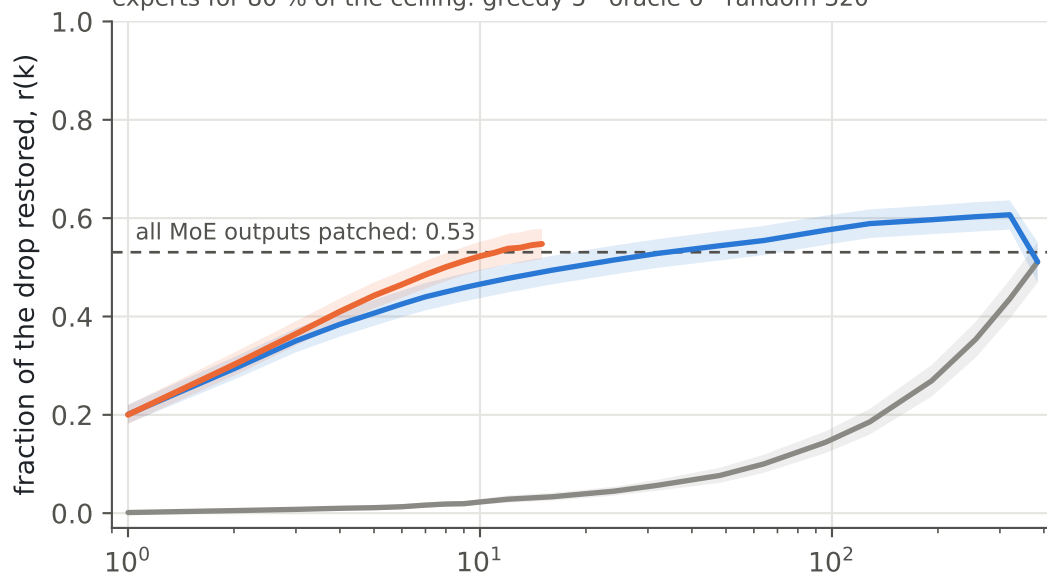
WinoGrande · Qwen3-30B-A3B (K = 384)
