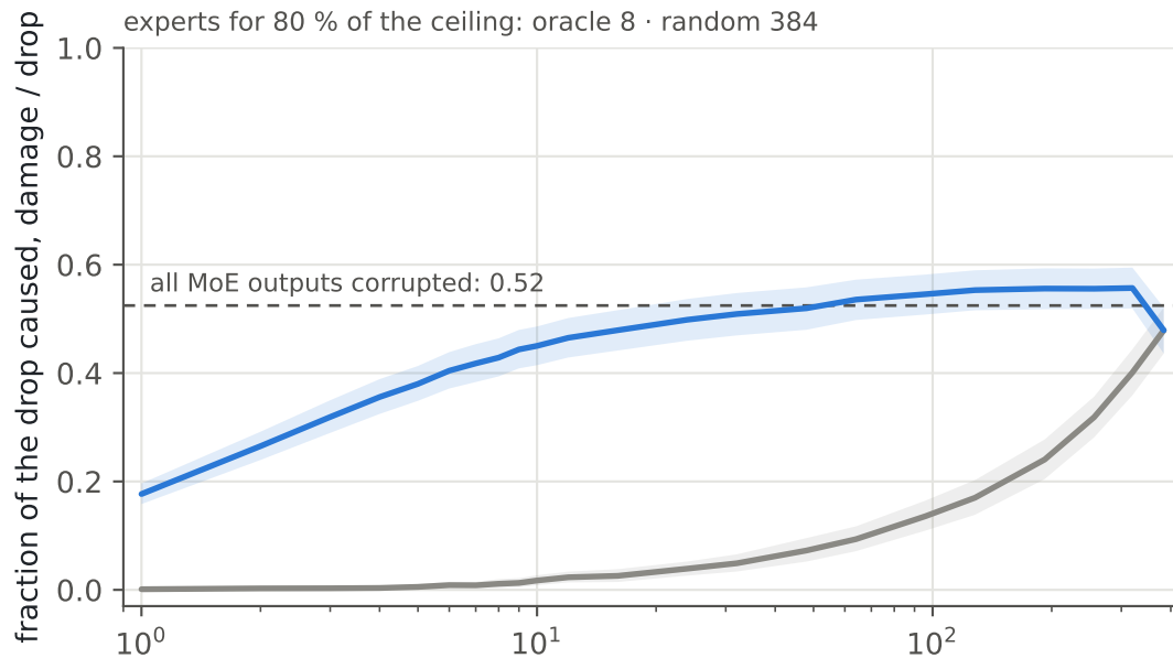
WinoGrande · Qwen3-30B-A3B (K = 384)
