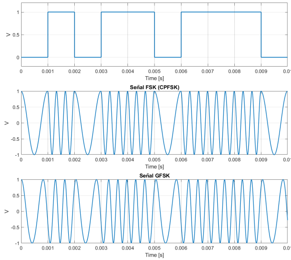
Figura 7: Comparación entre señales NRZ, FSK y GFSK (BLE).
