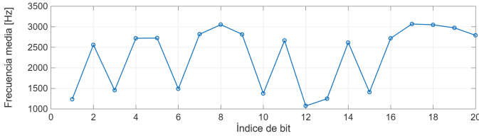
Figura 10: Frecuencia instantánea promedio por intervalo de bit obtenida durante el proceso de demodulación GFSK
