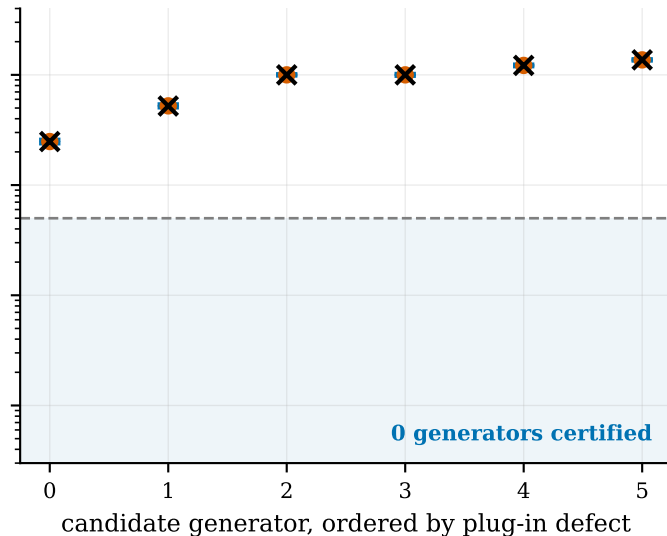
(b) Van der Pol: none
