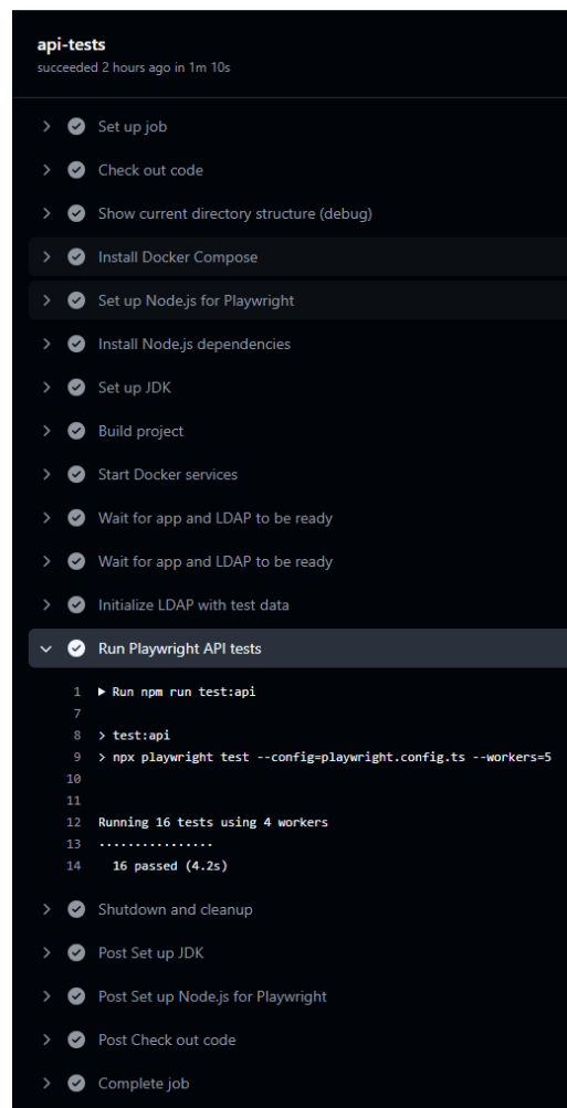
Abbildung 13.10: Erfolgreicher Playwright-Testlauf innerhalb der CI/CD-Pipeline
