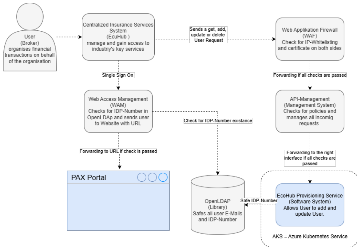
Abbildung 9.5: C2-Diagramm IST-Zustand - Containerübersicht (Quelle: Eigene Darstellung)
