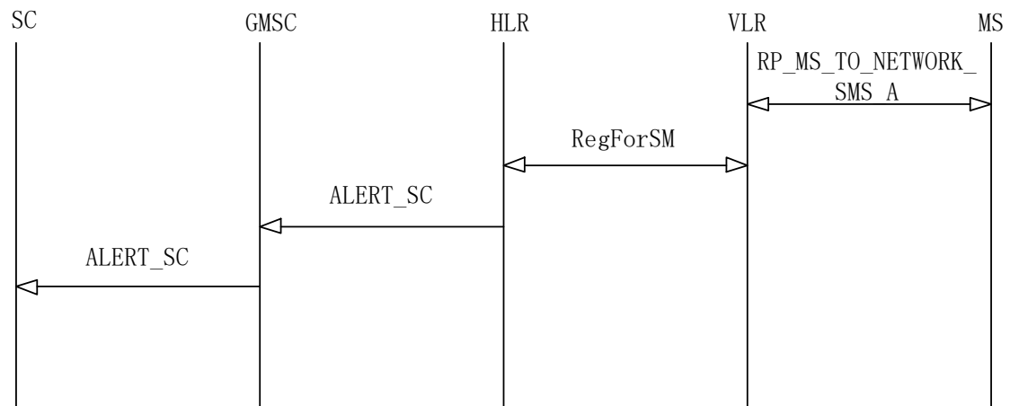
图 3-17 Alert-SC 信令流程
