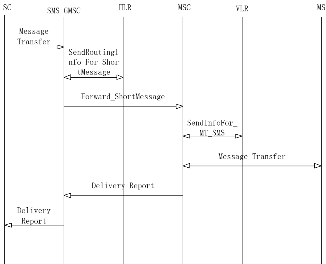
图 3-16 MT 信令流程
