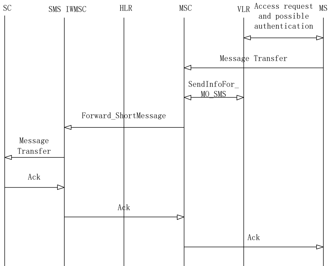
图 3-15 MO 信令流程
