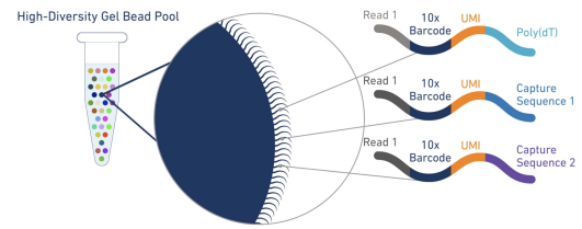
Fig. 1. Schéma explicatif de la technique de séquençage d'ARNm sur cellules uniques (credit : 10xGenomics)
