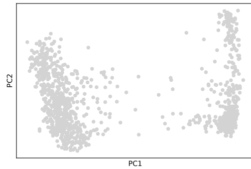
Fig. 10. ACP en 2 dimensions : méthode 2
