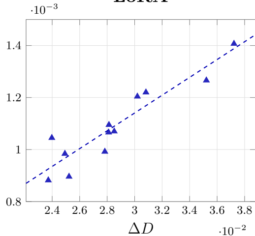
LoRA
