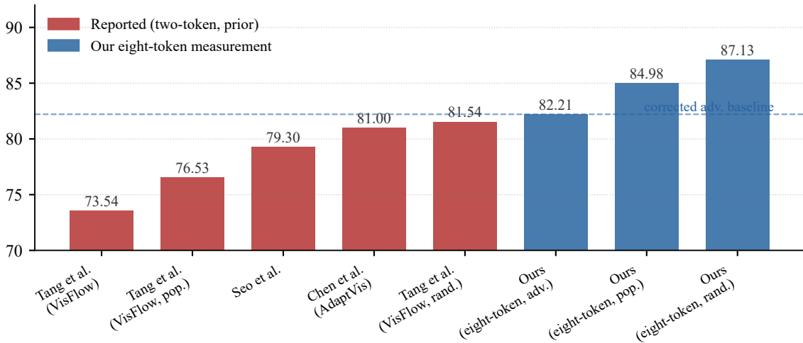
POPE F1 (x100)
