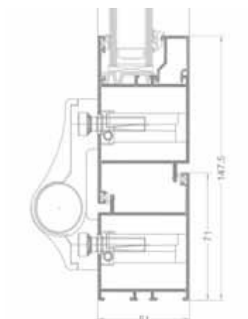
ŘEZ DVEŘE
