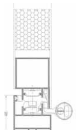
ŘEZ PANELOVÉ DVEŘE
