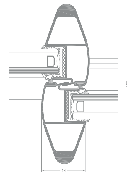
řez spojením křídlo-křídlo
