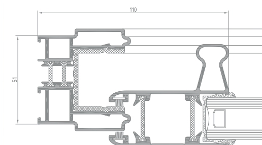
řez dveřmi SL+
