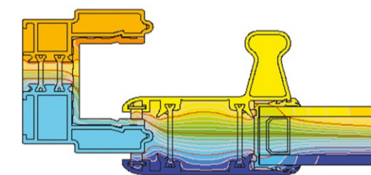
příklad rozložení izoterm v sestavě rámu a křídla SLIDE PLUS (SL 010 + SL 1120)
