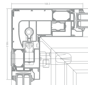
řez pohyblivým rohovým sloupkem UG
