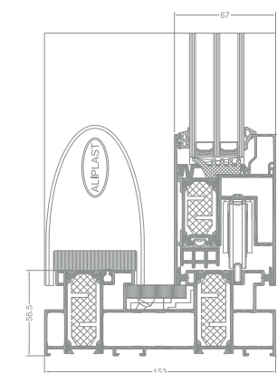
UG řez rámem a křídlem (UG 820 + UG 810)
