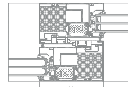
Řez spojením křídlo-křídlo (UG 820 + UG 830)
