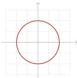
\|\mathbf{v}\|_2 = 1 : a circle
