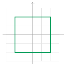
\|\mathbf{v}\|_\infty = 1 : a square
