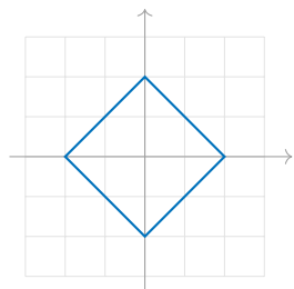
\|\mathbf{v}\|_1 = 1 : a diamond
