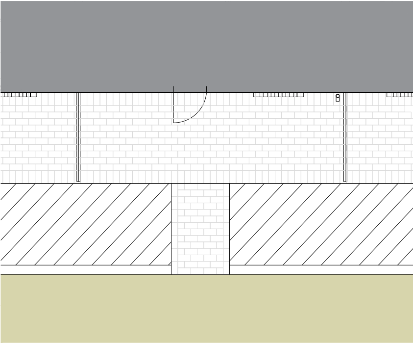
PRINCIP MÖNSTERLÄGGNING BETONGMARKSTEN P4
