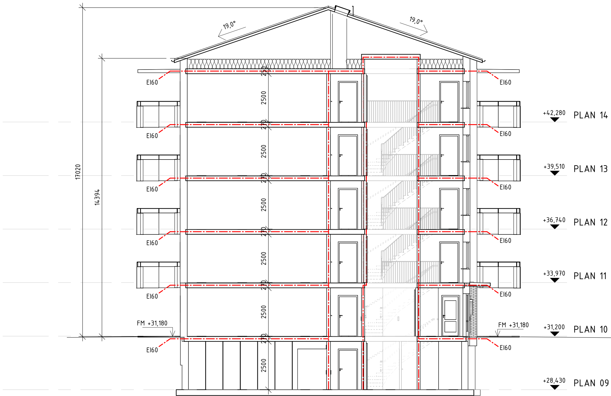
SEKTION A-A
