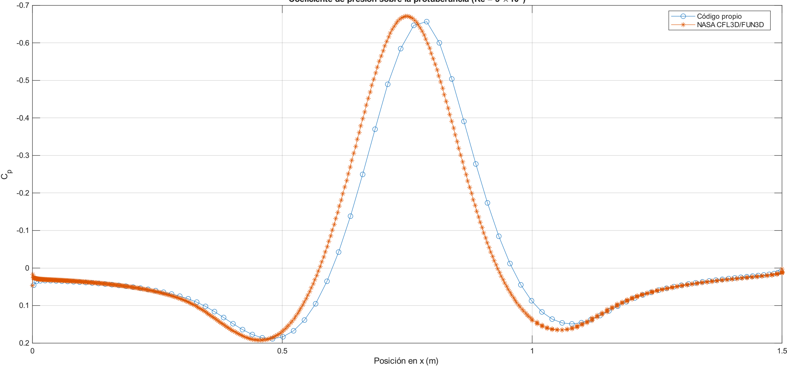
Coeficiente de presión sobre la protuberancia ( Re = 3 \times 10^6 )
