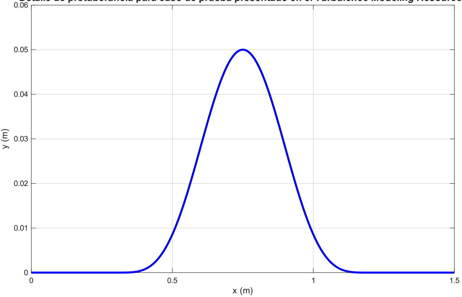
Detalle de protuberancia para caso de prueba presentado en el Turbulence Modeling Resource
