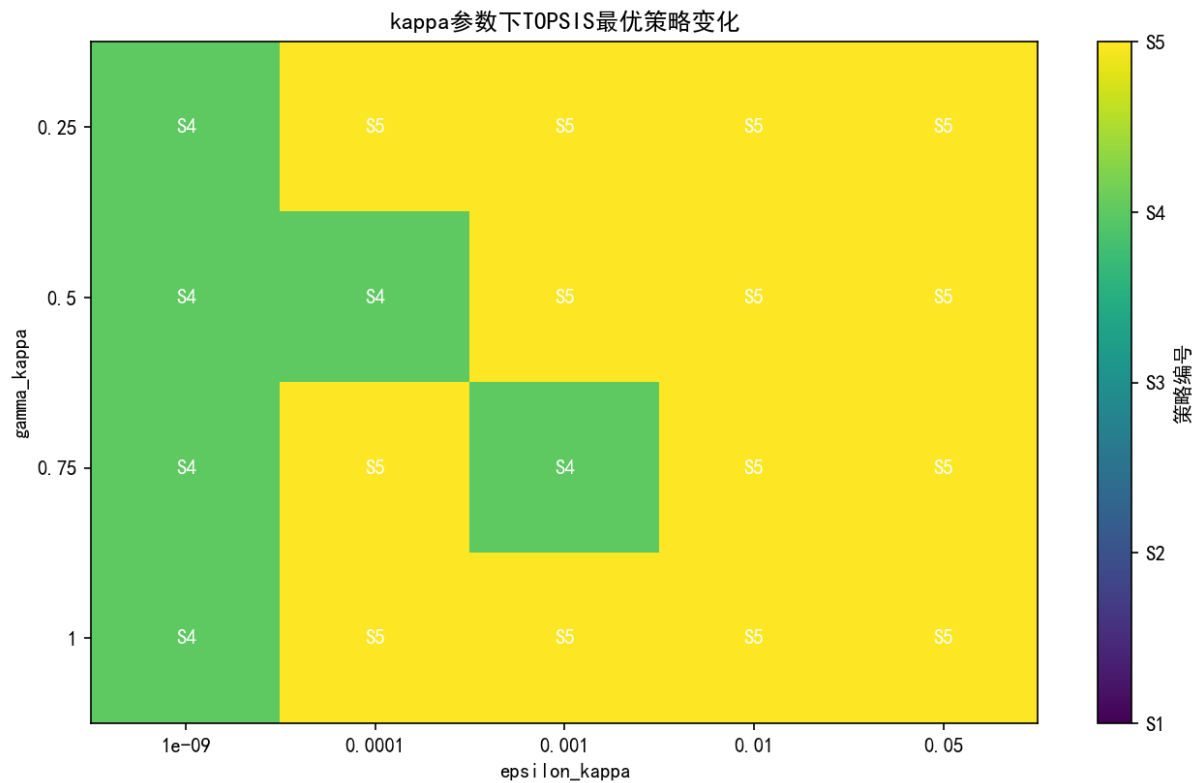
图 16 \kappa 参数下最优策略变化热力图。不同 \gamma_\kappa 和 \epsilon_\kappa 组合会影响 S4、S5 的最优策略归属；S5 在多数短期 \kappa 情景中综合排序更高，但 S4 的利润差为正情景更多。
