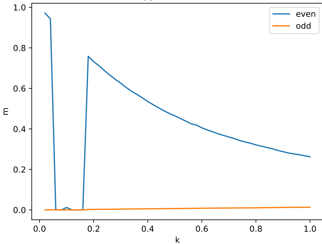
scipyGaussian,d=2
