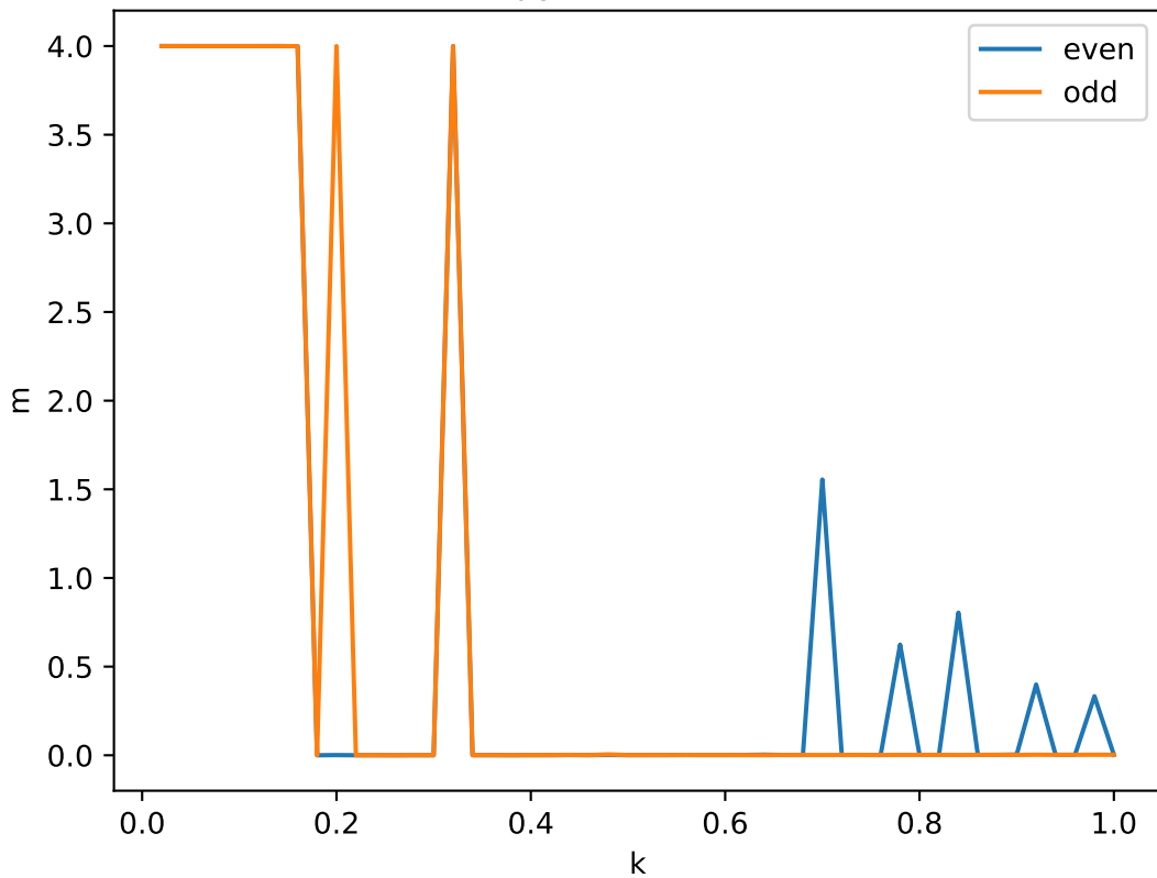
scipyGaussian,d=4
