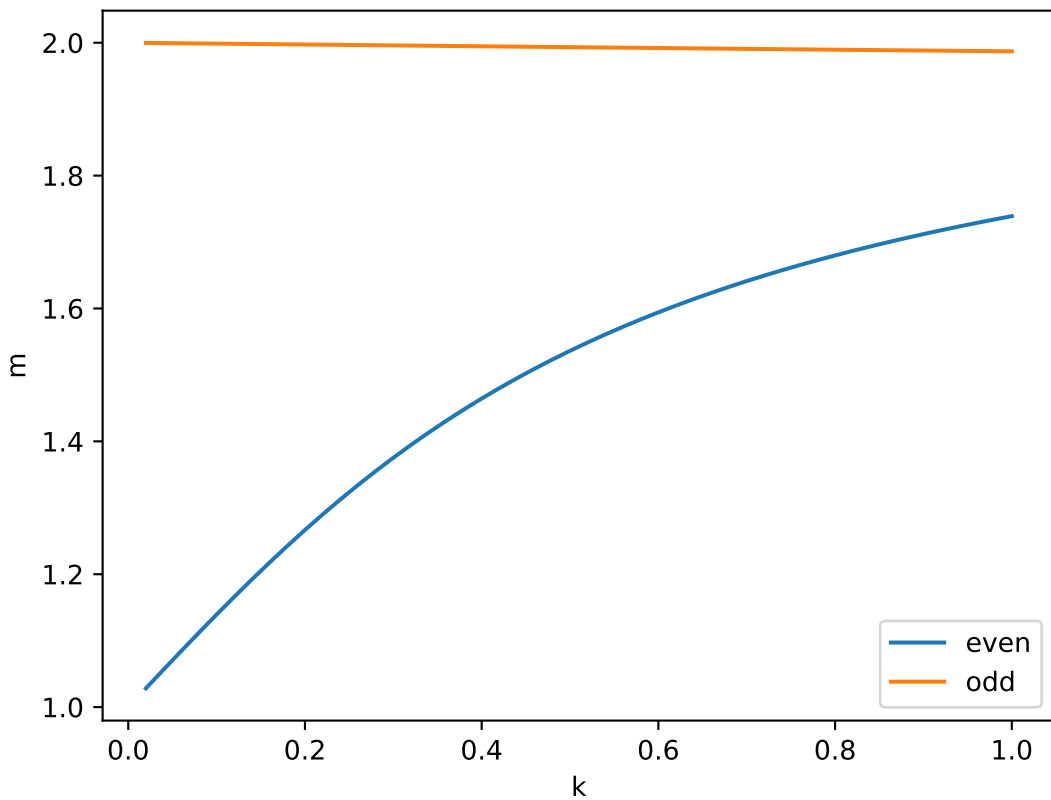
testGaussian,d=2
