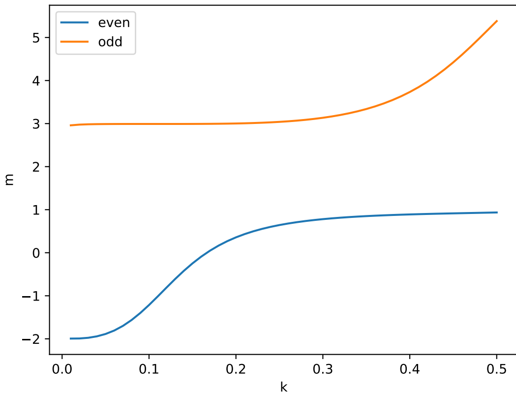
testGaussian,d=8
