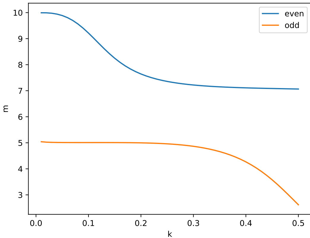
testGaussianReverse,d=8
