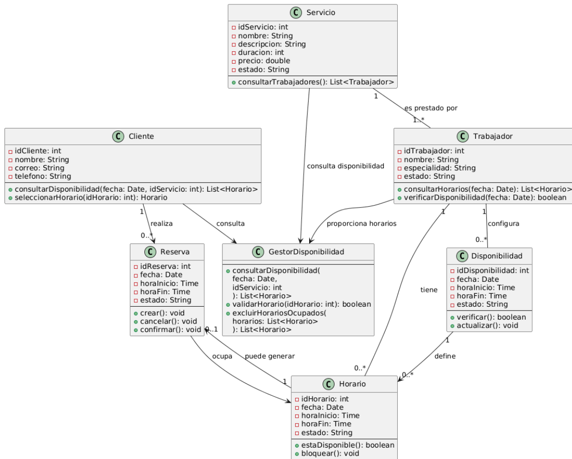
Diagrama de Clases - Visualizar Horarios de Trabajadores Disponibles
