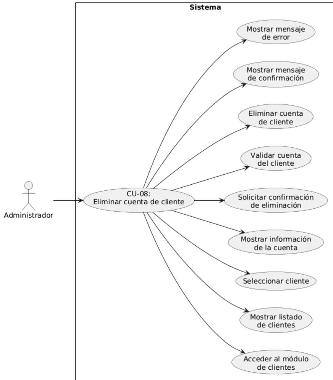
Diagrama de caso de uso - RF-08 Eliminar cuenta de cliente
