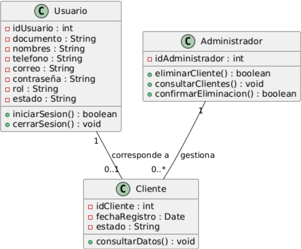
Diagrama de Clases - RF-08 Eliminar cuenta de cliente
