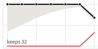
MiniMax-M2.5
