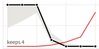
DeepSeek-V4-Flash
