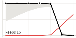
gemma-4-31B
