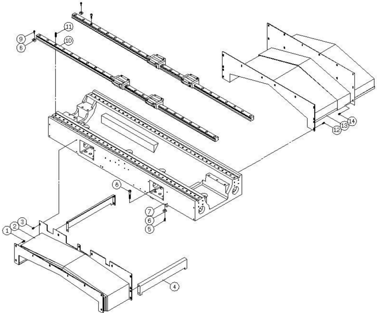
Baugruppe Schlitten - Carriage Assembly
