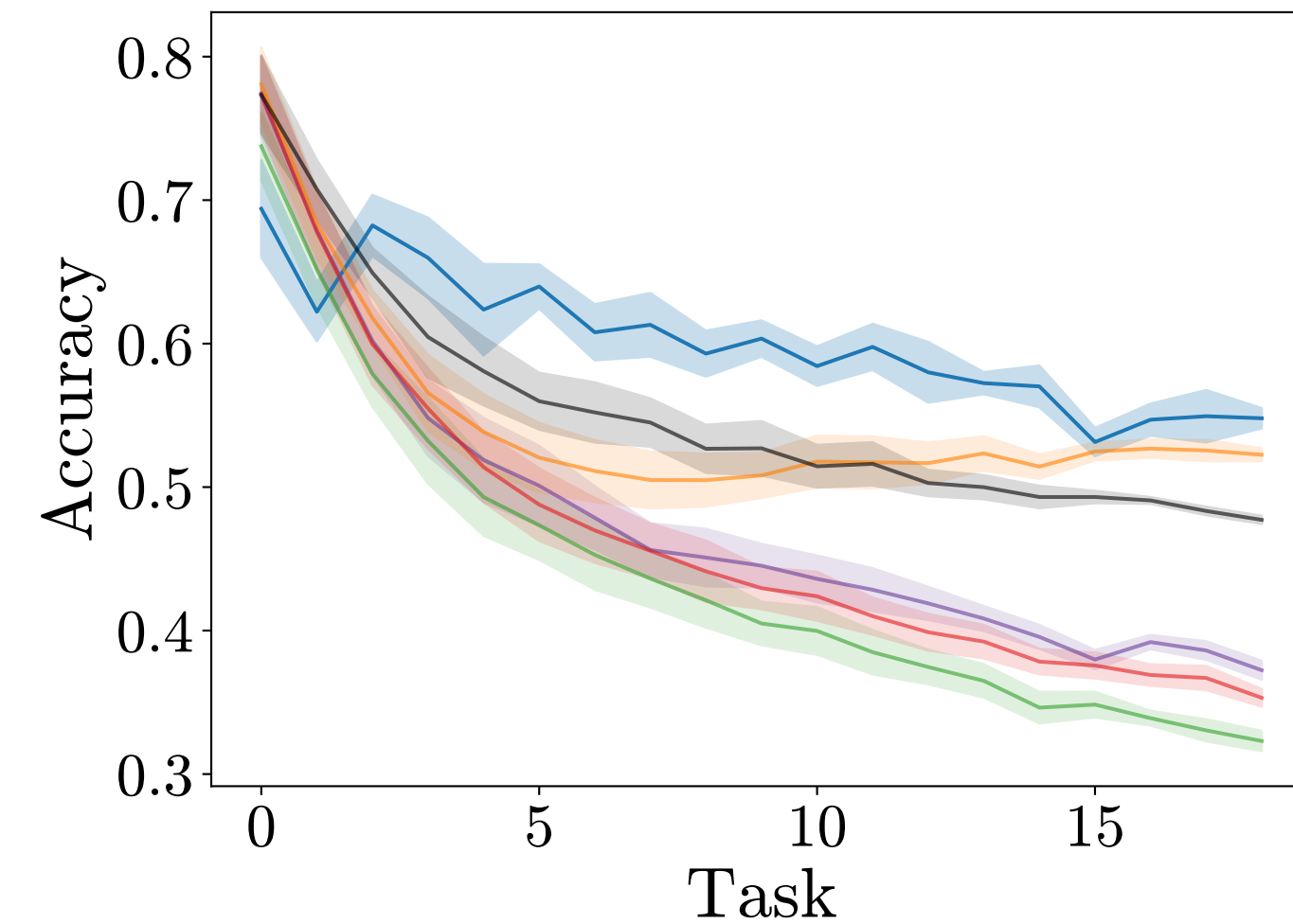
Incremental CIFAR
