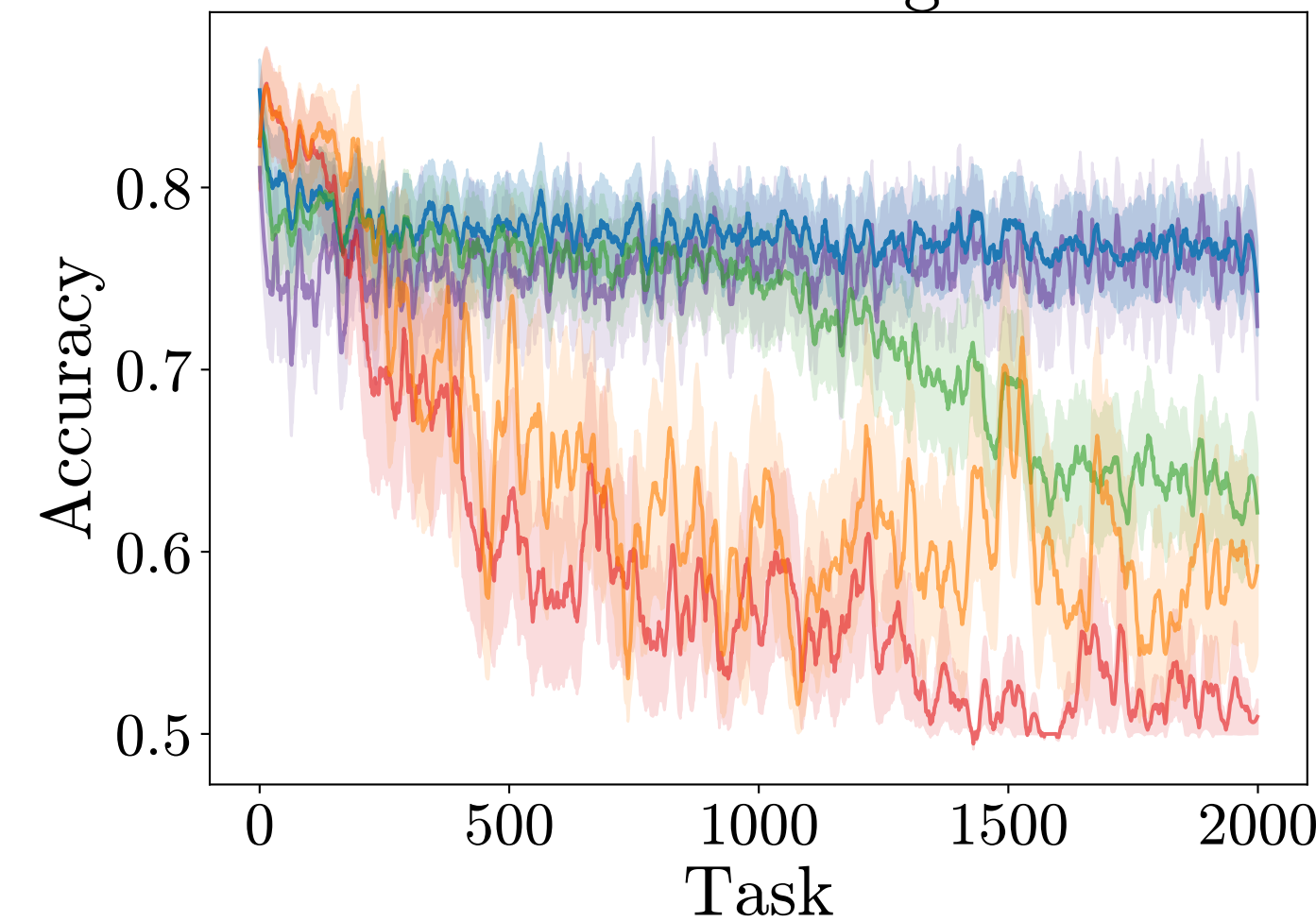
Continual ImageNet
