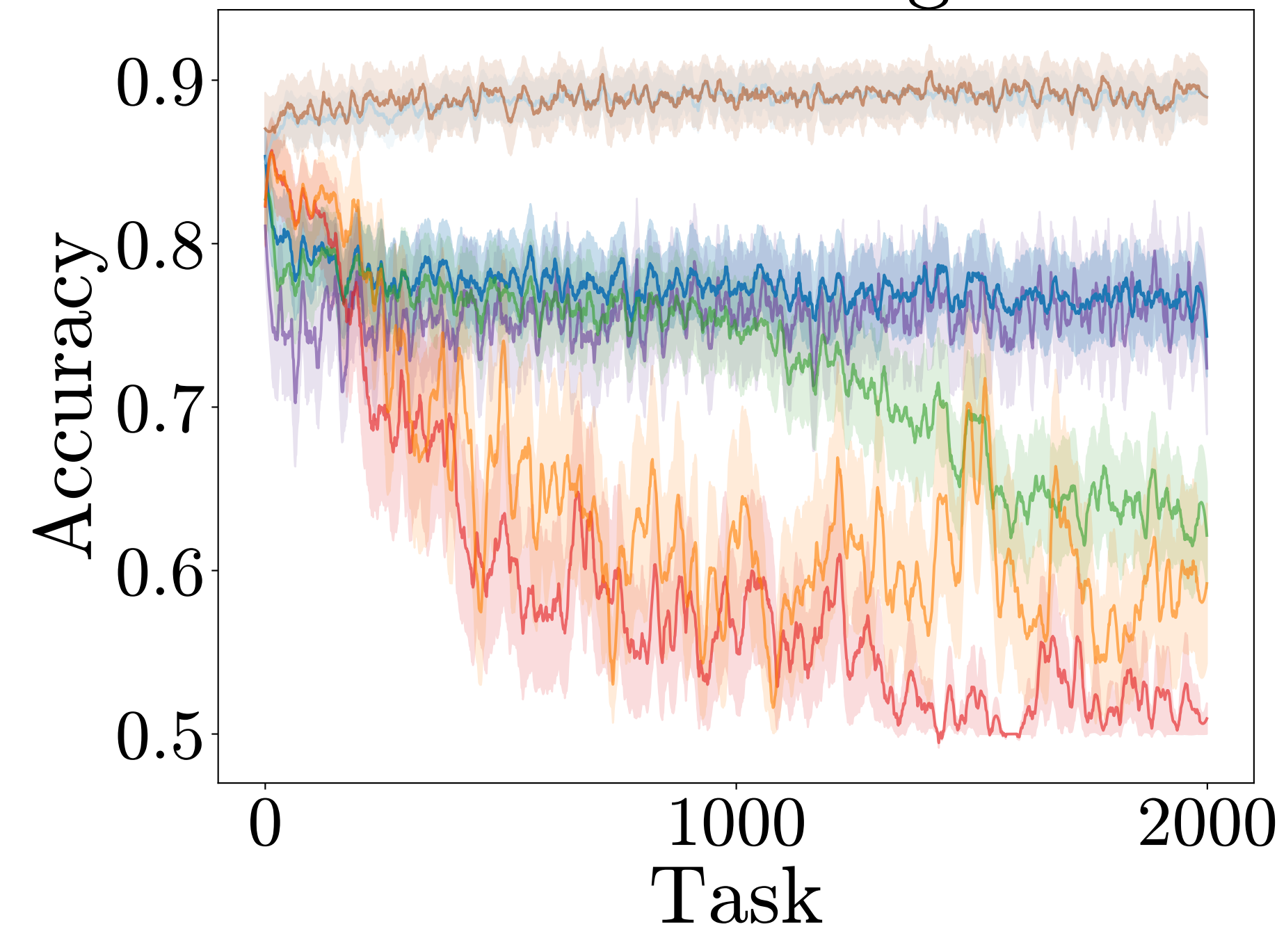
Continual ImageNet
