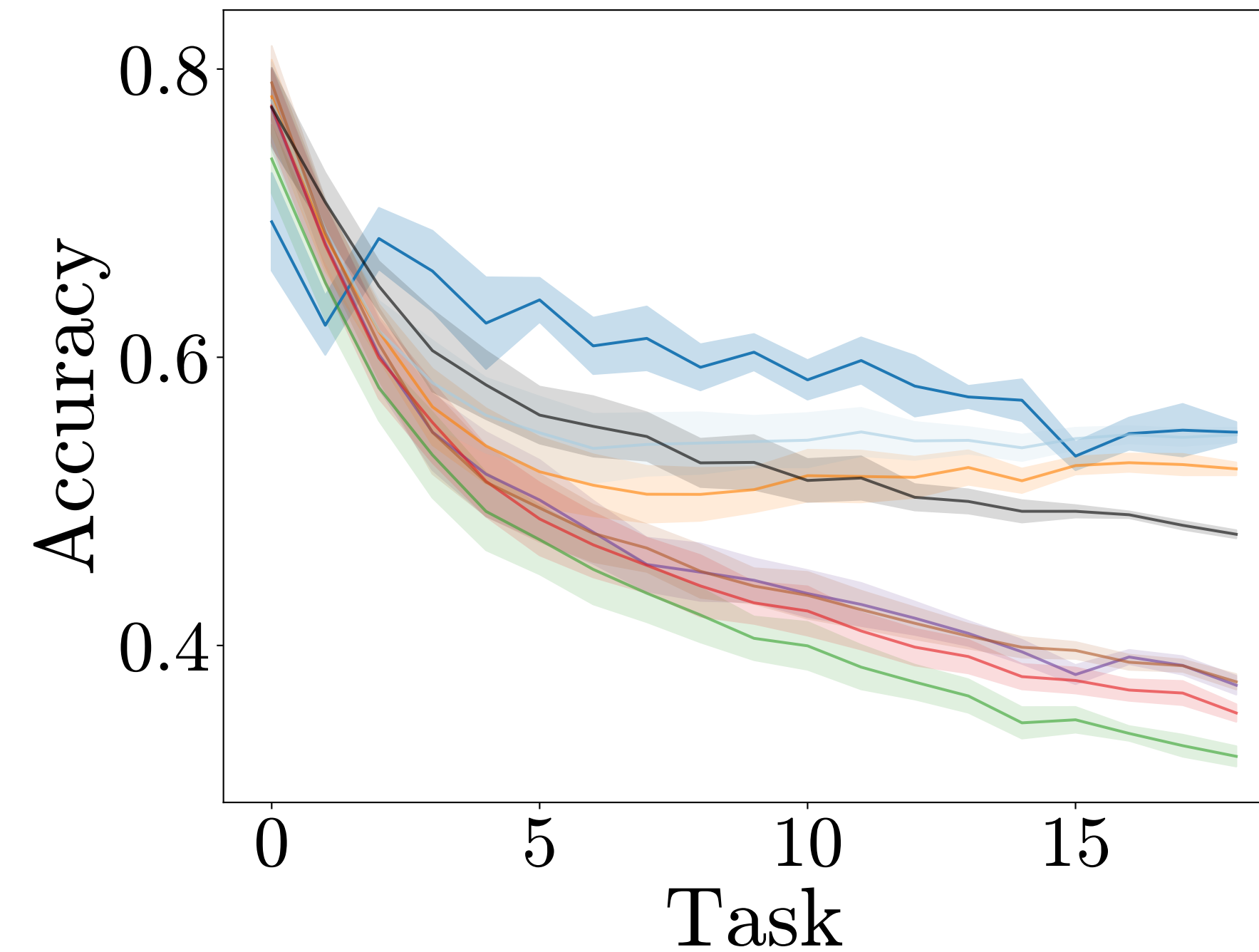
Incremental CIFAR
