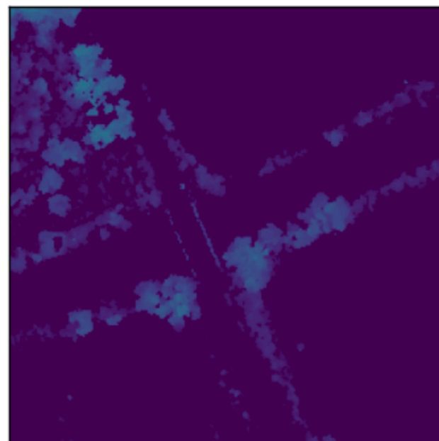
LiDAR GT
