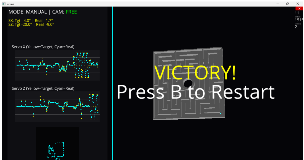
Figura 2: Interface em tela dividida exibindo a dinâmica 3D, gráficos de telemetria do PD e histórico de trajetória.
