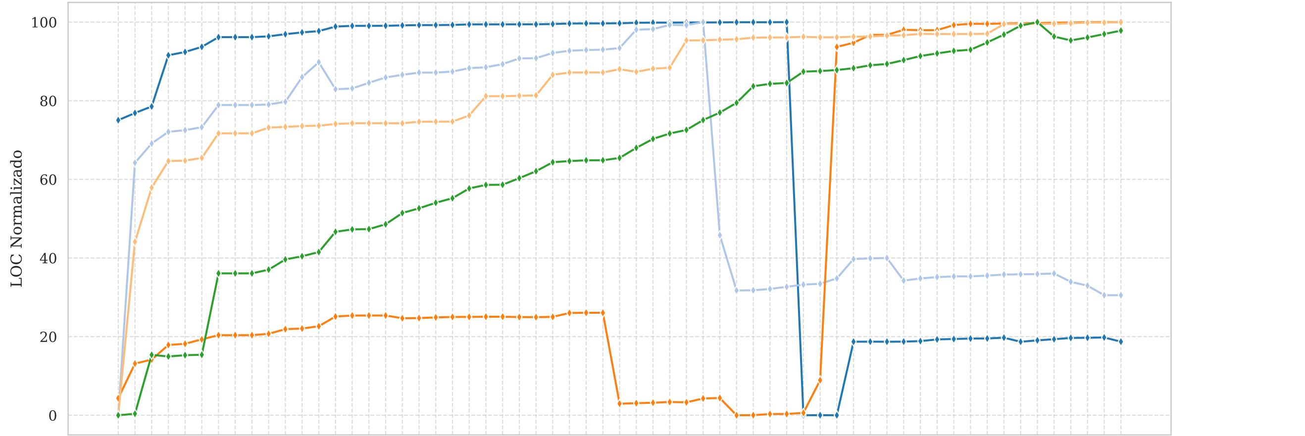
Média de LOC por Método Ativo (Grandes: Início > 500k LOC)
