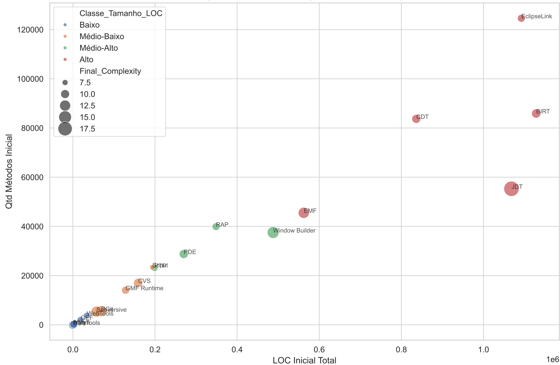
Tamanho Inicial: LOC vs Quantidade de Métodos (Tamanho da bolha = Complexidade LOC/Método)
