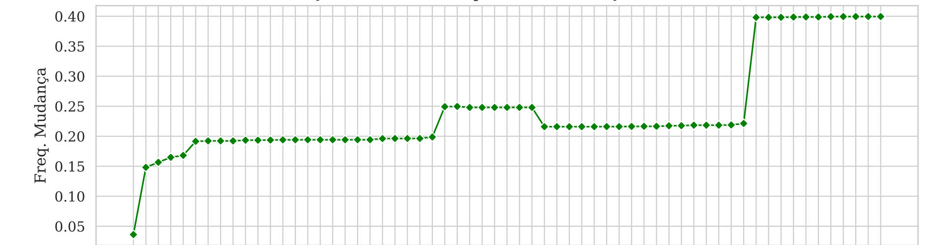
Evolução - WebTools - Frequência de Mudança (FRCH Médio)
